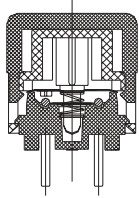
Part N° shown: 5T52-S2x
